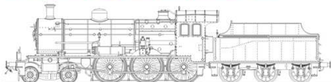
Vanaf 1918 plaatsing voorverwarmer en ombouw ganghandel naar rechts
